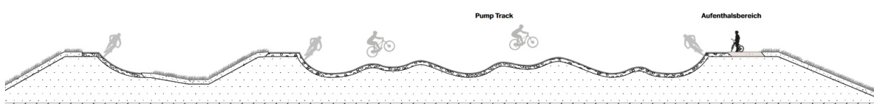
Schnitt B - B Massstab 1:250
