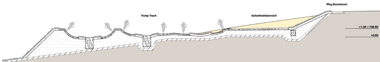
Schnitt A - A Massstab 1:250
